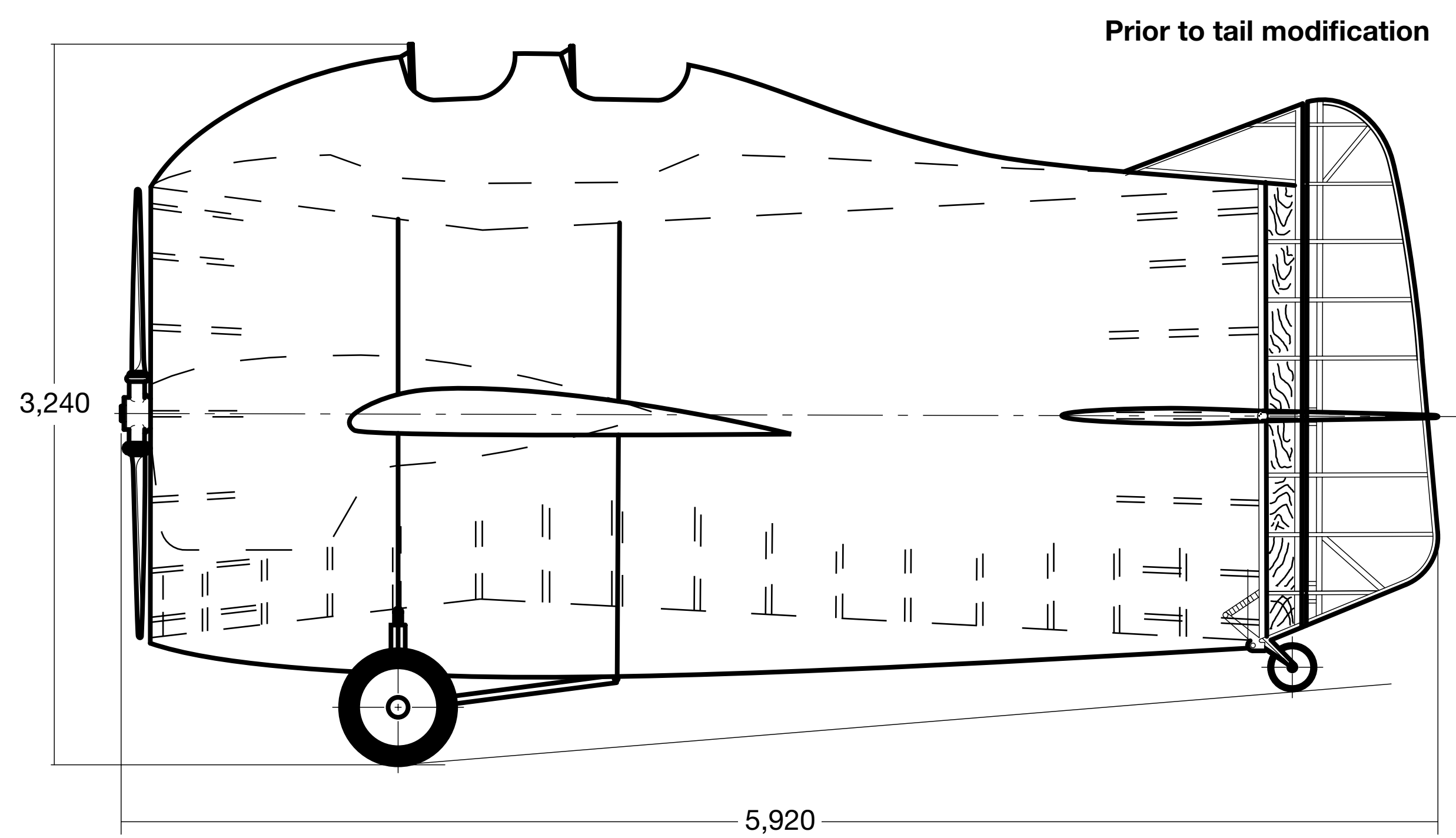
Stipa-Caproni Insieme Schemarico - Vista di Fianco Side View with Schematic Scale 1/20
